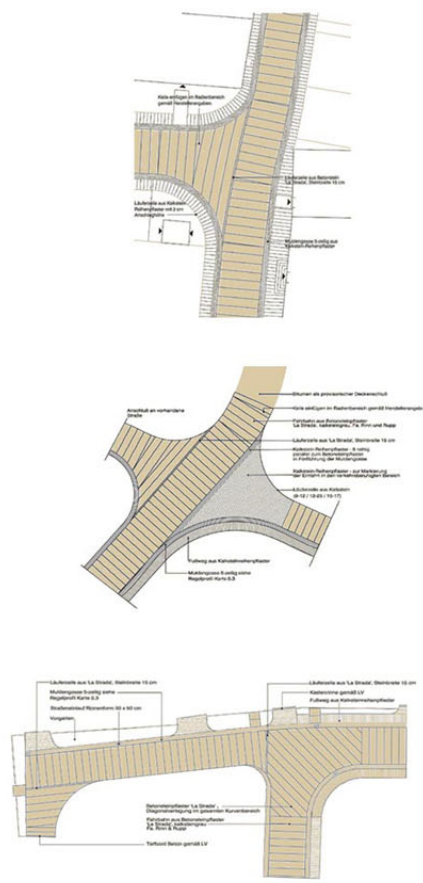
Pflasterdetails
